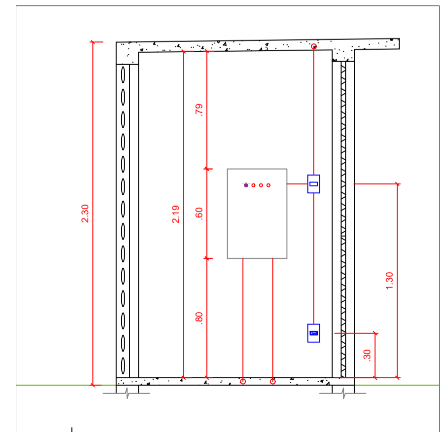
CORTE 1-1 ESC.: 1/25
