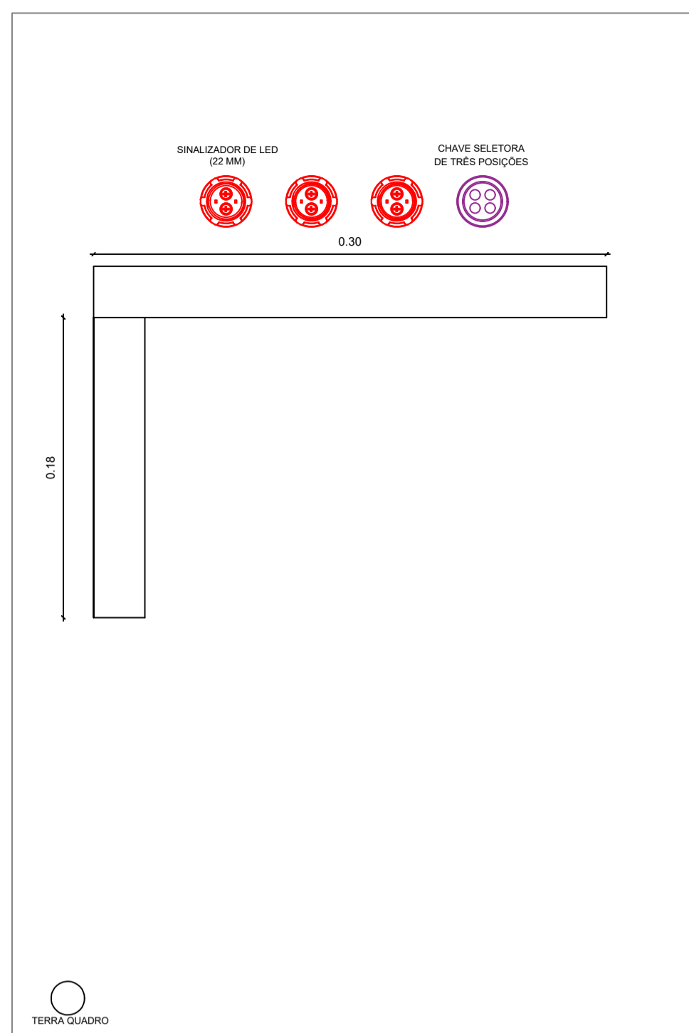
PORTA INTERNA - QUADRO GERAL DE COMANDO S/ESC.
