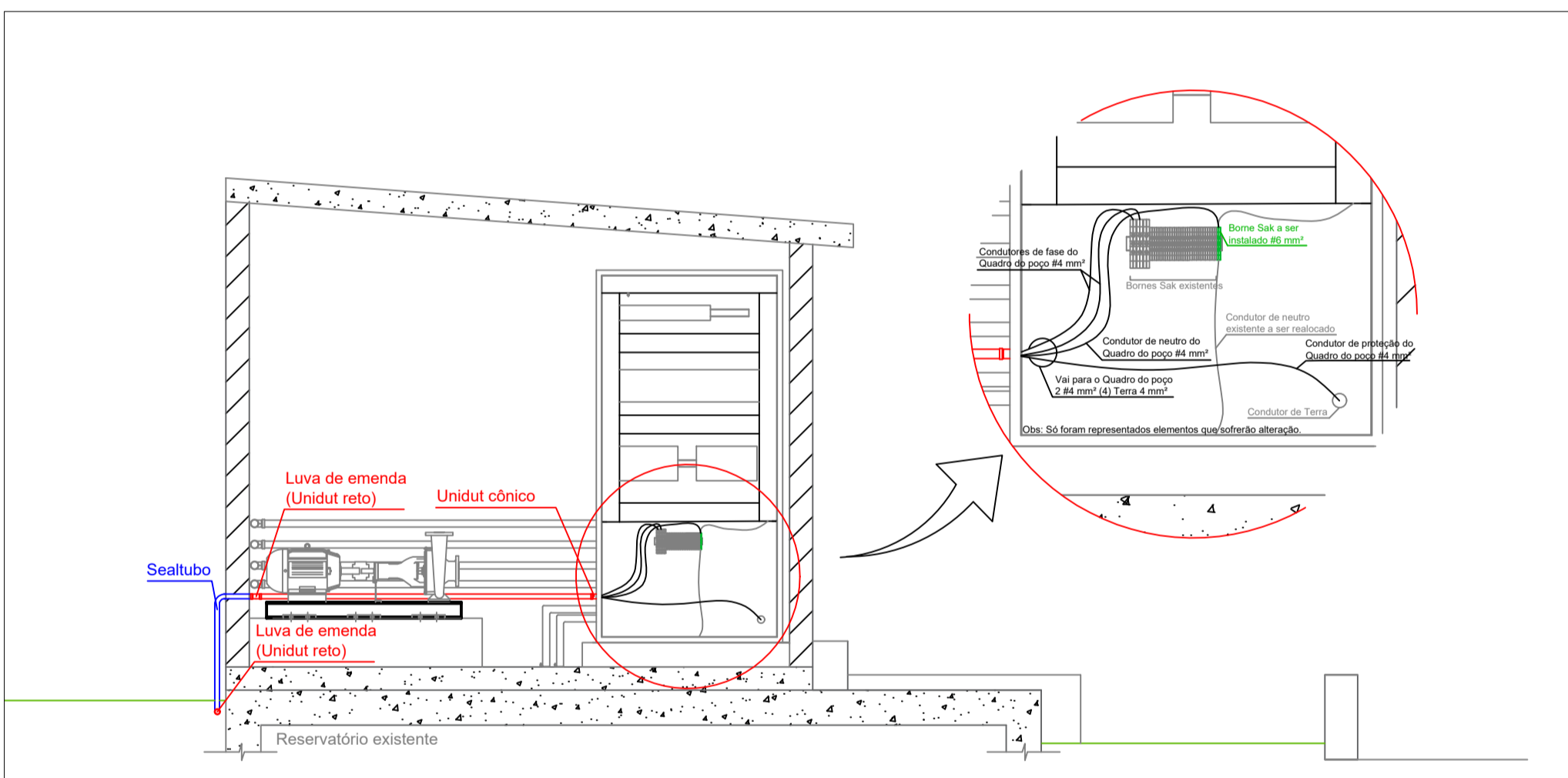
QUADRO DA CISTERNA - DETALHAMENTO ESC.: 1/25
