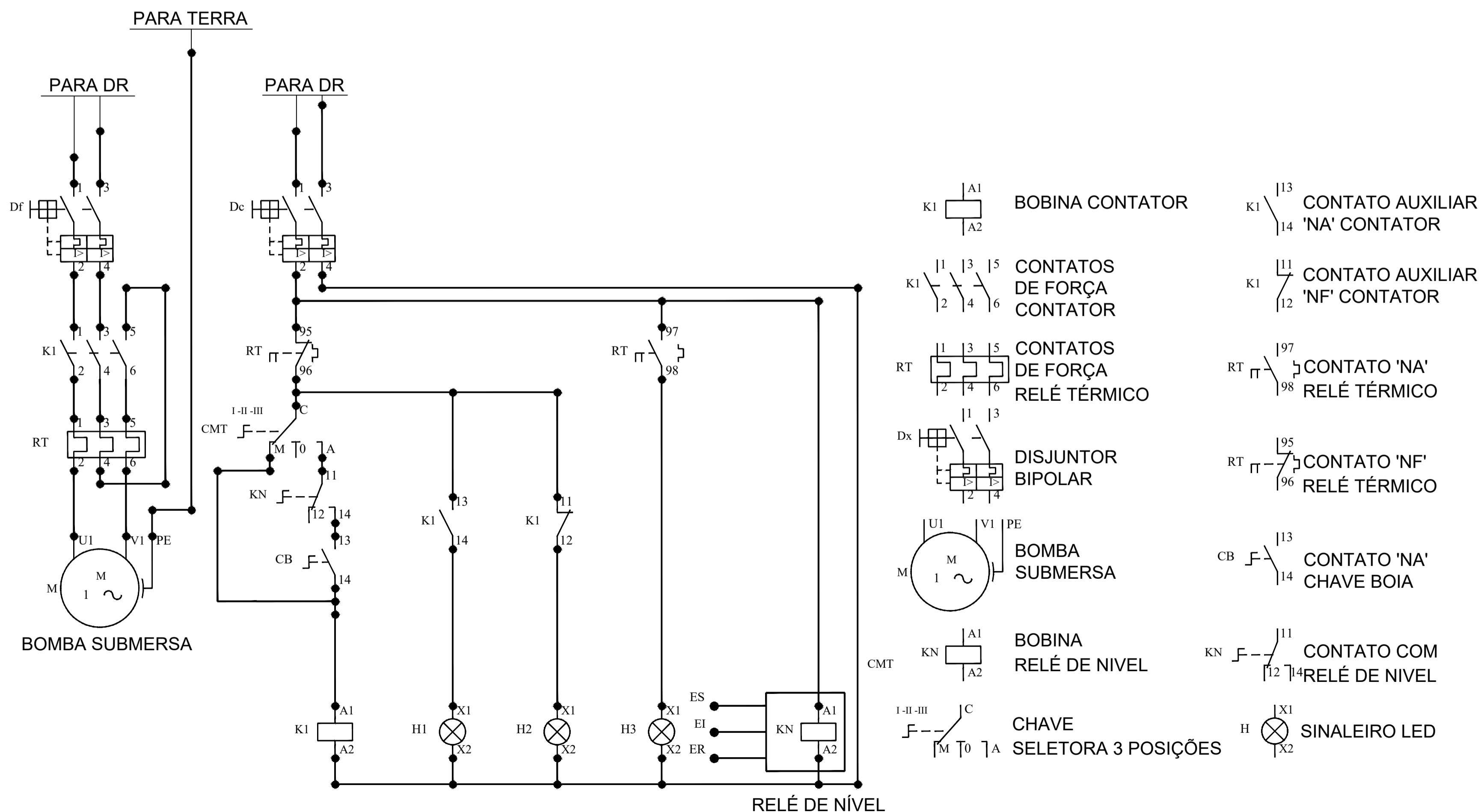
DIAGRAMA DE COMANDO S/ESC.
