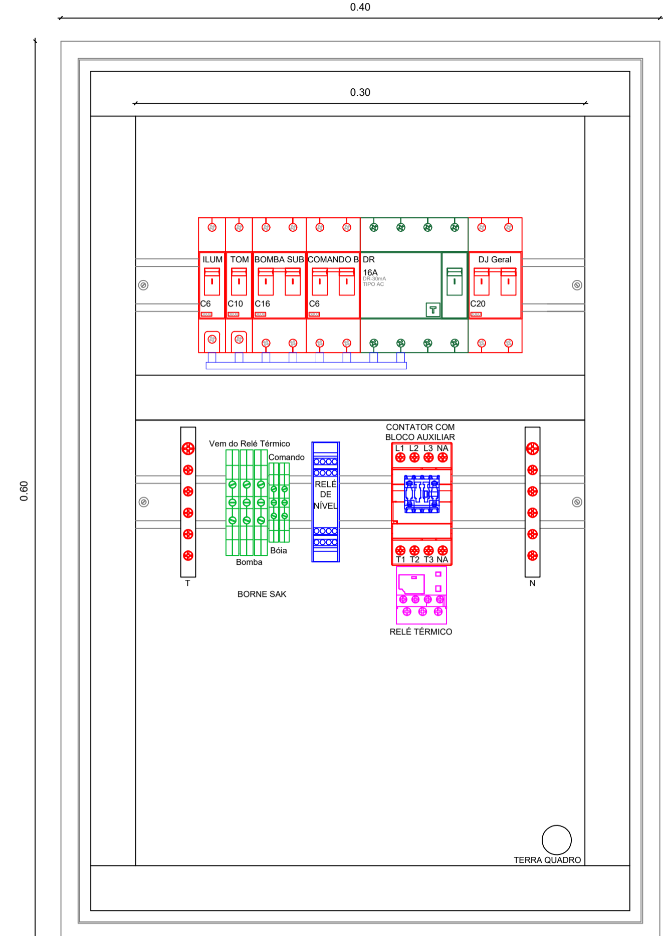
QUADRO GERAL DE COMANDO ESC.: 1/2
